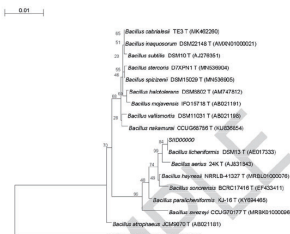
図1-1. SIID0000000の16S rDNA塩基配列に基づく簡易分子系統樹 左上の棒はスケールバー、系統樹の分岐に位置する数字はブートストラップ値、 株名の末尾のTはその種の基準株 (Type strain)、BSLはバイオセーフティレベル (BSL1:日常環境中に以上を育記) を示します。
