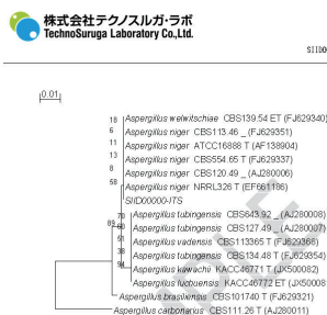
図1. rRNAのITS領域塩基配列に基づく糖基分子系統樹 左上の棒はスケールバー。系統樹の分岐に付随する数字はブートストラップ値、枝名の末尾の 括弧内は両側の念珠球上のタイプの種数である。*はスペース(空白)を示し、**は
